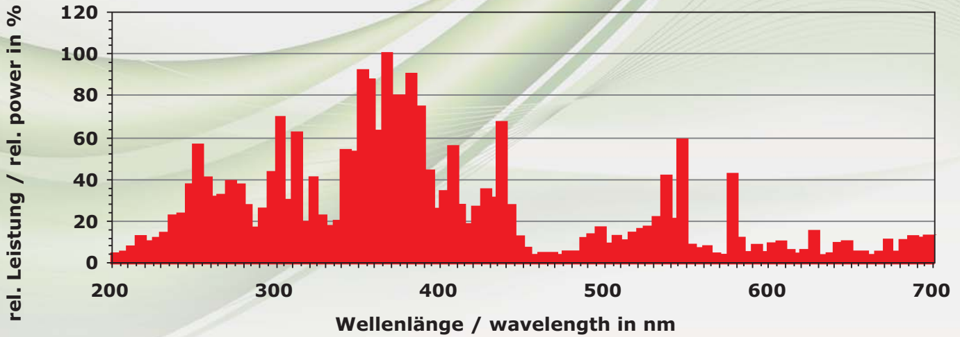
Spektrum UVH-Strahler, Typ Fe / Spectrum UVH-lamp, type Fe (Eisen dotiert / iron doped)
